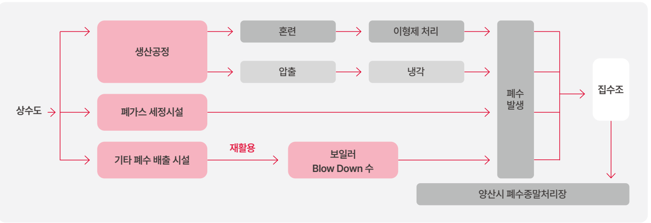
[E3-11] DRB오토모티브 폐수 처리 계통도
