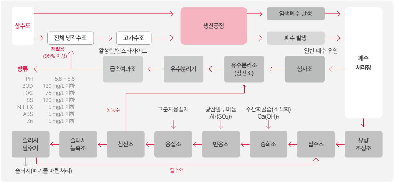
[E3-10] 동일고무벨트 폐수 처리 계통도
